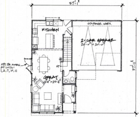
FIRST FLOOR SCALE: 1/8" = 1'-0"
